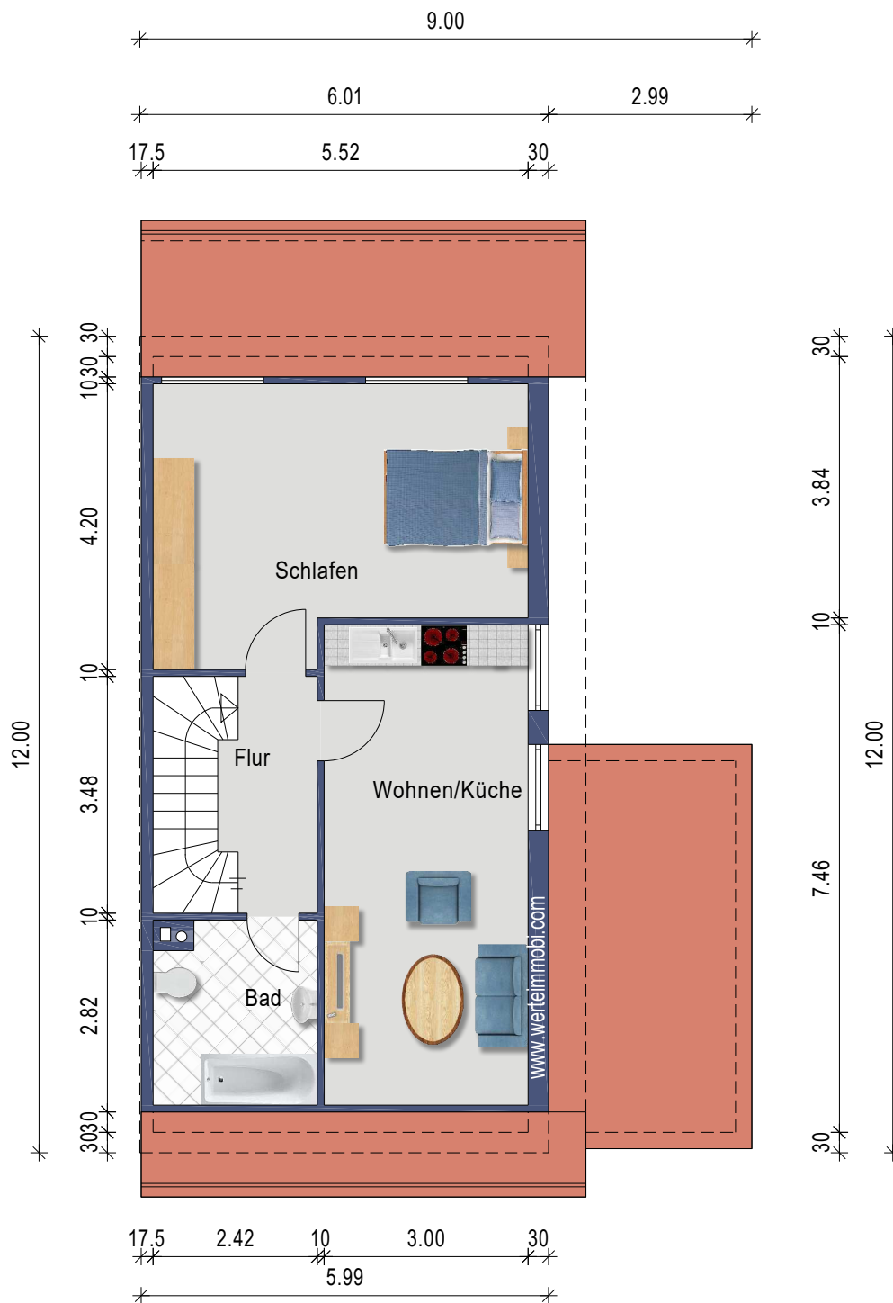
Dachgeschoss
