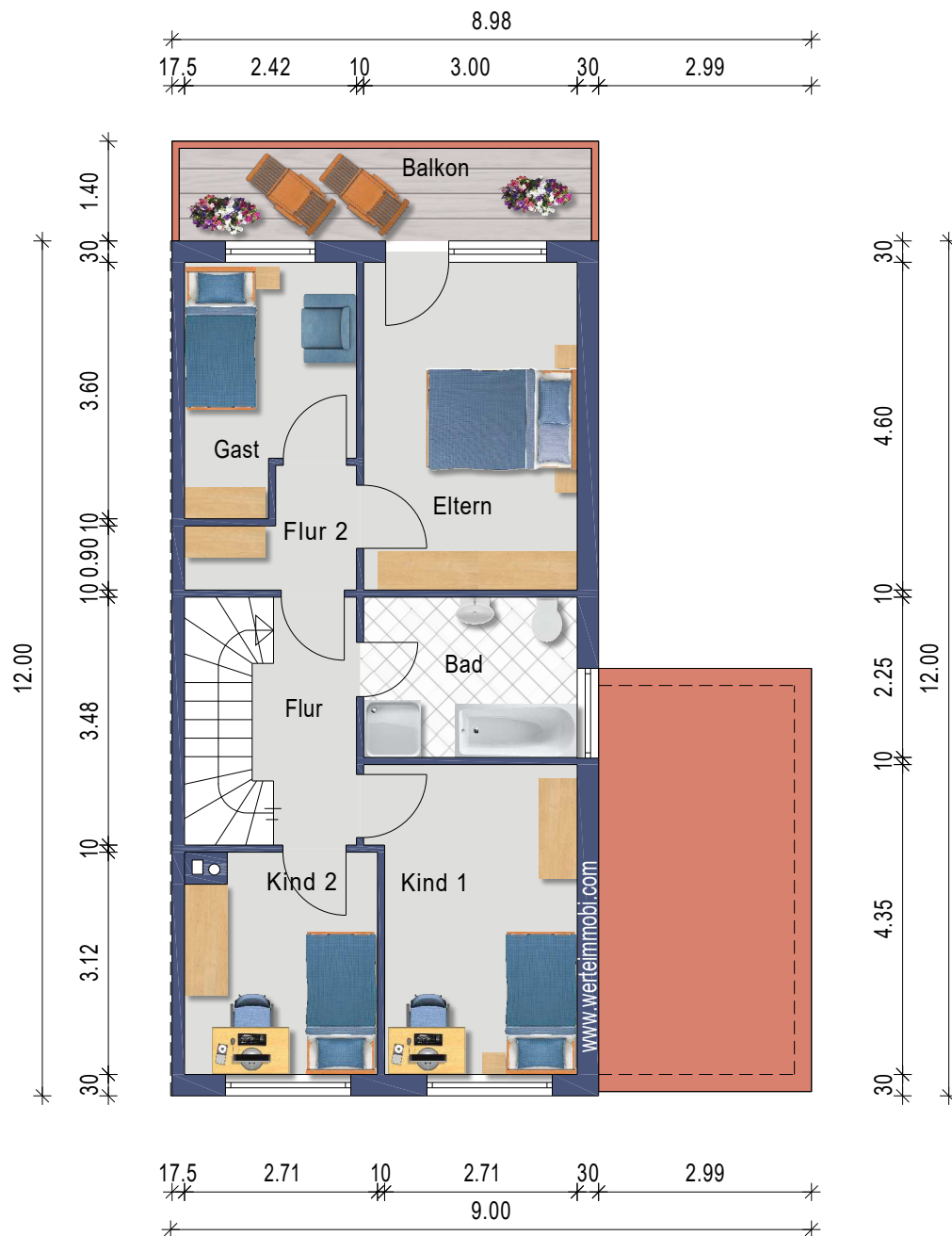
Obergeschoss
